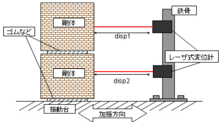
図 1 変位計測例
