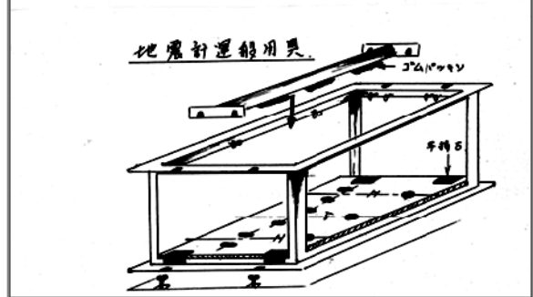
● 宮崎観測所：勝島短周期地震計移動用具
