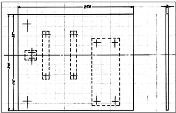
● 伸縮計センサー部：ステンレス基板配置図
