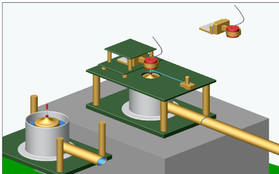
●センサーフロート：回転防止機能
