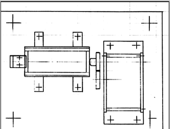
● 宮崎観測所坑道：立坑伸縮計スライド部
