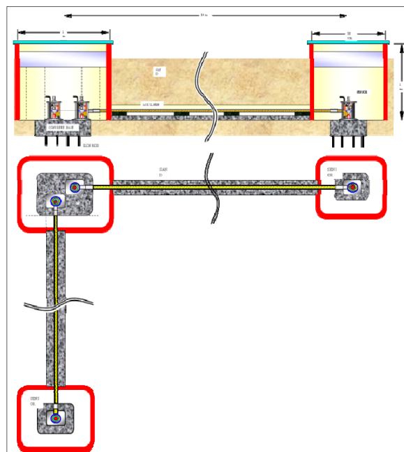
● インドネシアオイル傾斜計全体図
