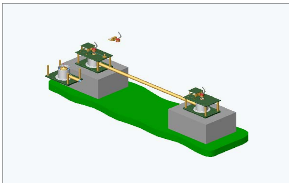
● Ver2でのフルフィールド水管傾斜計全体図
