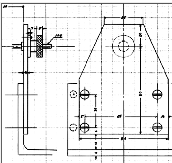
● 宮崎観測所坑道：立坑伸縮計センサー部
