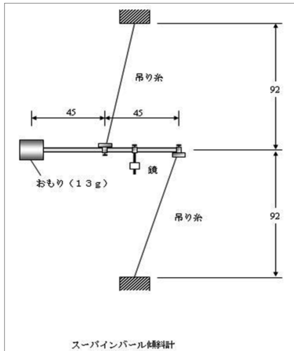
● スーパーインバル線傾斜計：振子部
