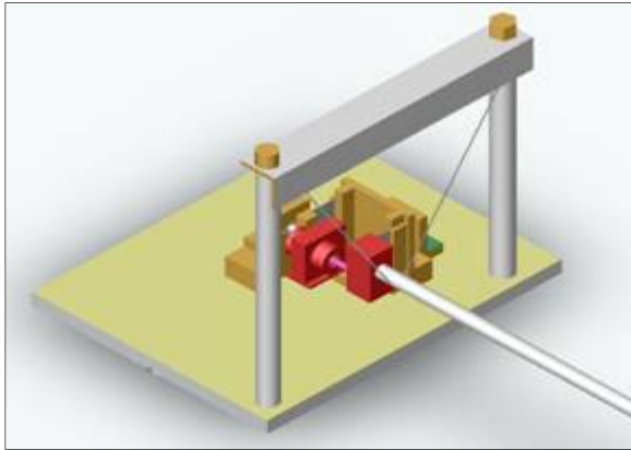
● 3D：由良観測室：スーパーインバール棒伸縮計
