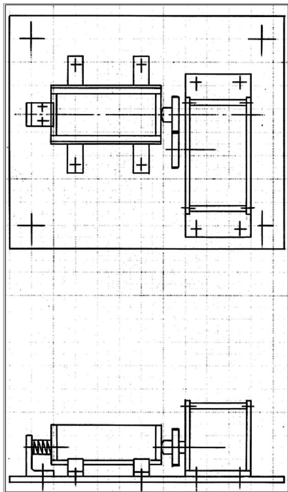
● 伸縮計センサー部全体側面図
