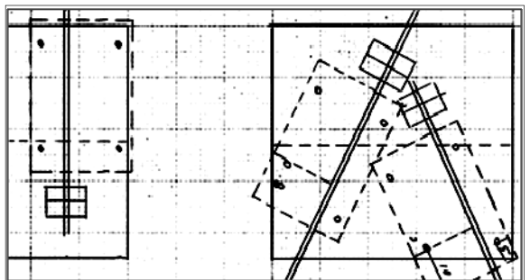
● 槇峰観測室坑道：伸縮計基礎台基板配置図
