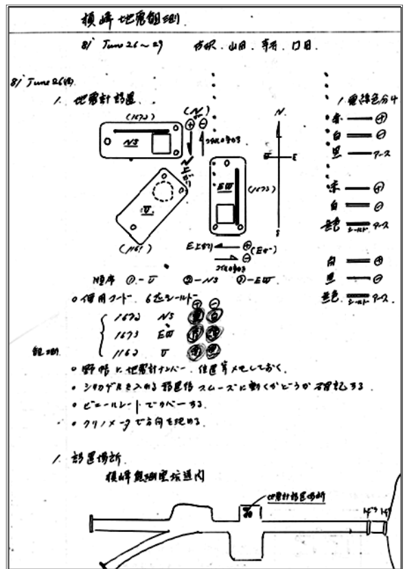
● 槇峰観測室坑道：短周期地震計設置場所
