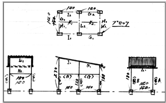
● 槇峰観測室坑道：観測計器用屋根全体図
