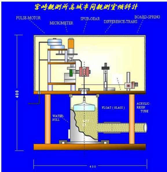
● フルフィールド 型水管傾斜計：センサー部
