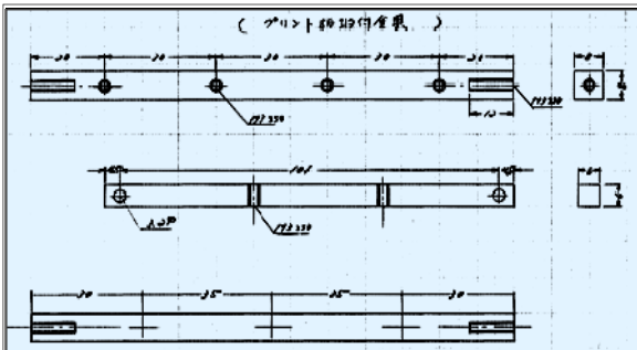
● アンプケース用固定金具
