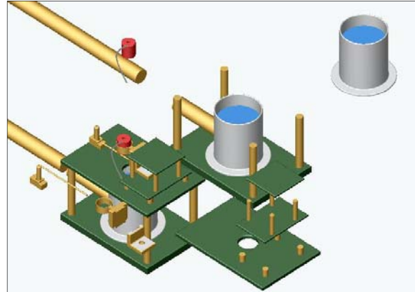
● 水管傾斜計拡大図：フルフィールド型 (II)
