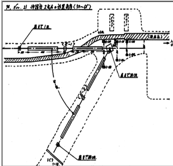
● 槇峰観測室坑道：伸縮計設置 60 度の場合
