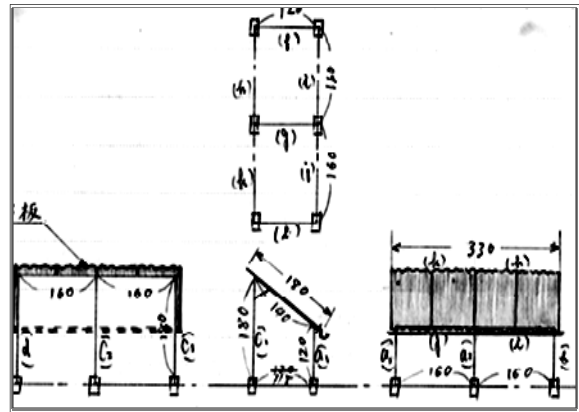
● 槇峰観測室坑道：観測計器用屋根全体図
