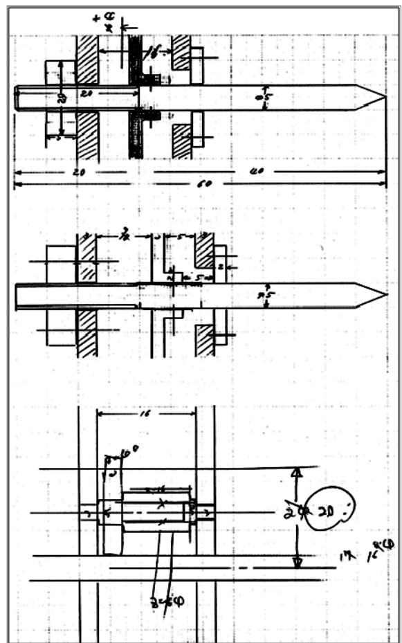
● 伸縮計調整用変速ギヤ試作品拡大
