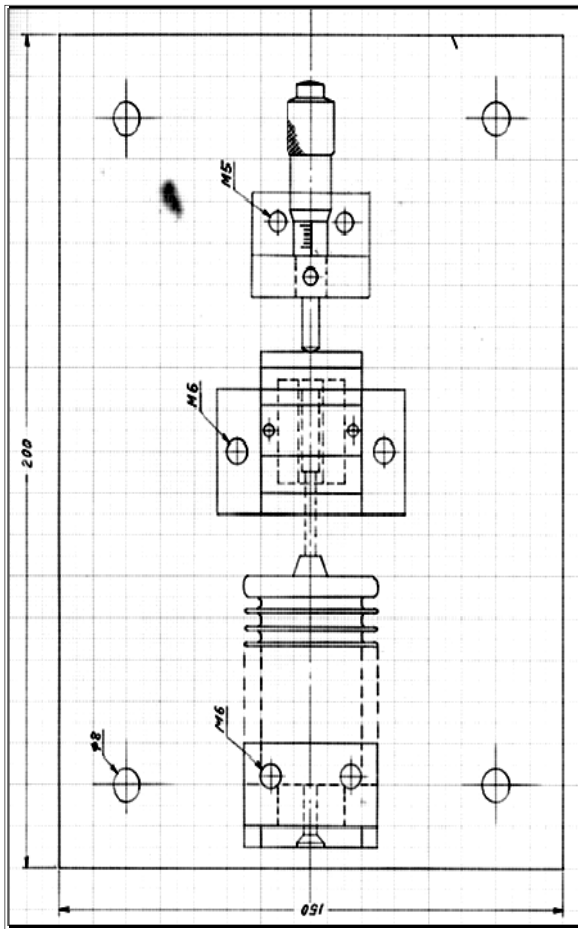
● 槇峰観測室坑道：ベローズ気圧計設計製作
