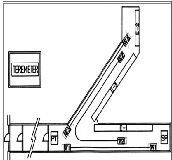
● 槇峰観測室坑道：地震地殻変動観測計器配置
