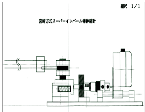
● スーパーインバル棒伸縮計：センサー部
