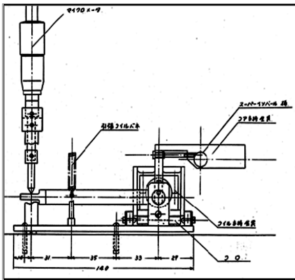
● 伸縮計センサー差動トランスマイクロ正面図
