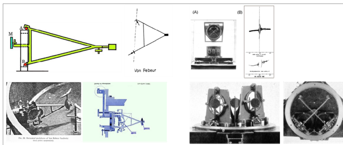
● 図1 構造原理と傾斜計写真
