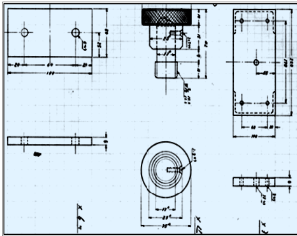
● 天ヶ瀬観測室坑道：光波測量基礎止め金具
