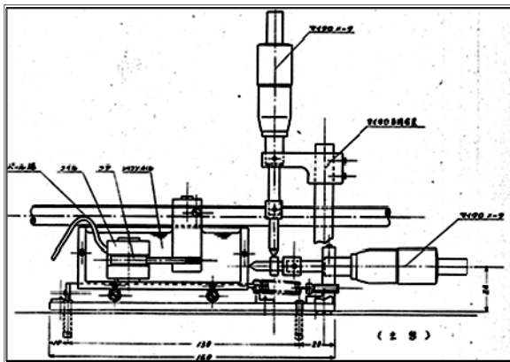
● 伸縮計センサー差動トランスマイクロ側面
