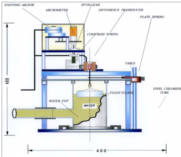
● 伊佐観測室坑道：水管傾斜計 2D 図
