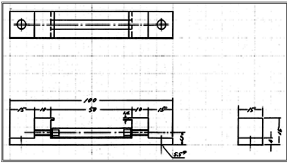
● 伸縮計センサー部：アクリルケース軸受
