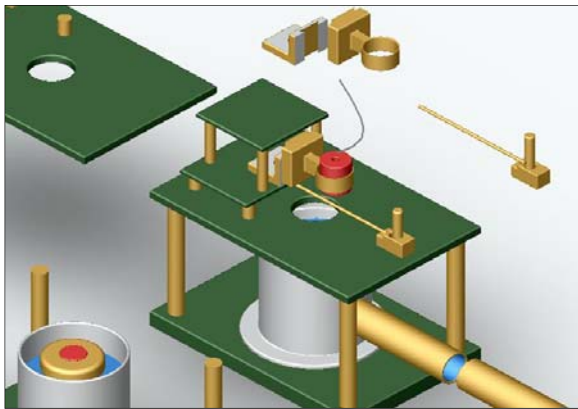
● 水管傾斜計拡大図：フルフィールド型 (I)
