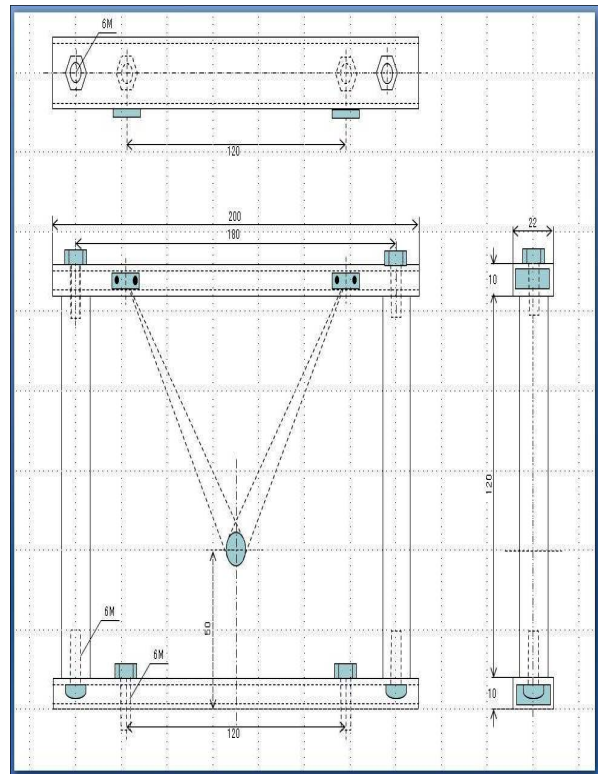
● スーパーインバール傾斜計吊り枠
