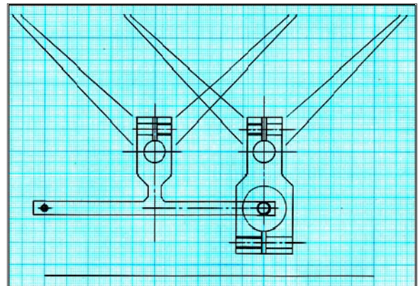
● 串間観測室：短周期地震計・傾斜計設置図
