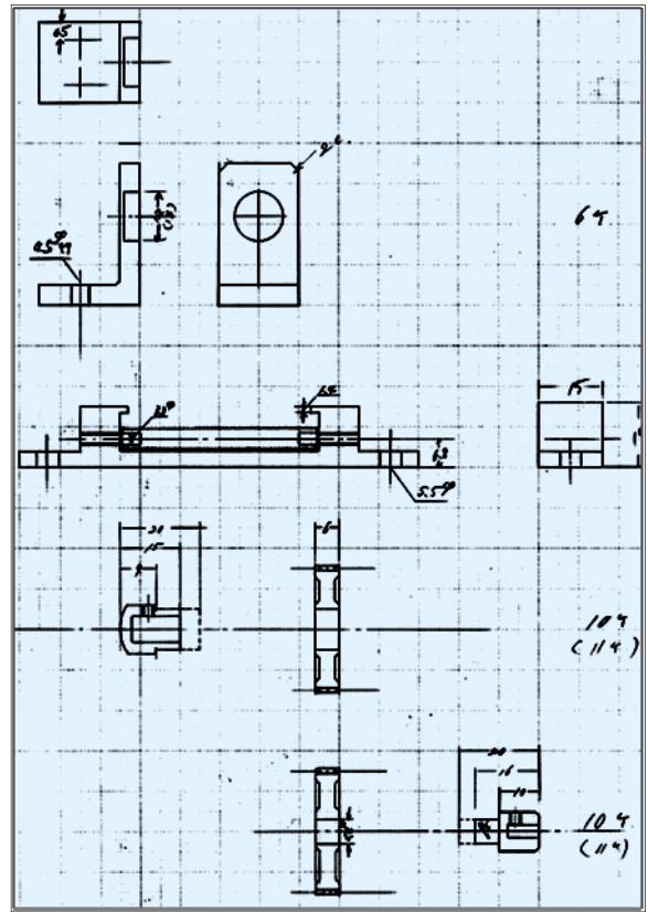
● 伸縮計センサー部：ケース軸受・歯車バネ受
