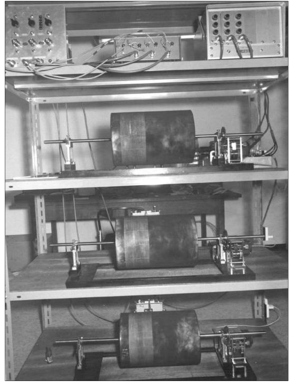
● 地震観測データ記録：煤書ドラム3成分
