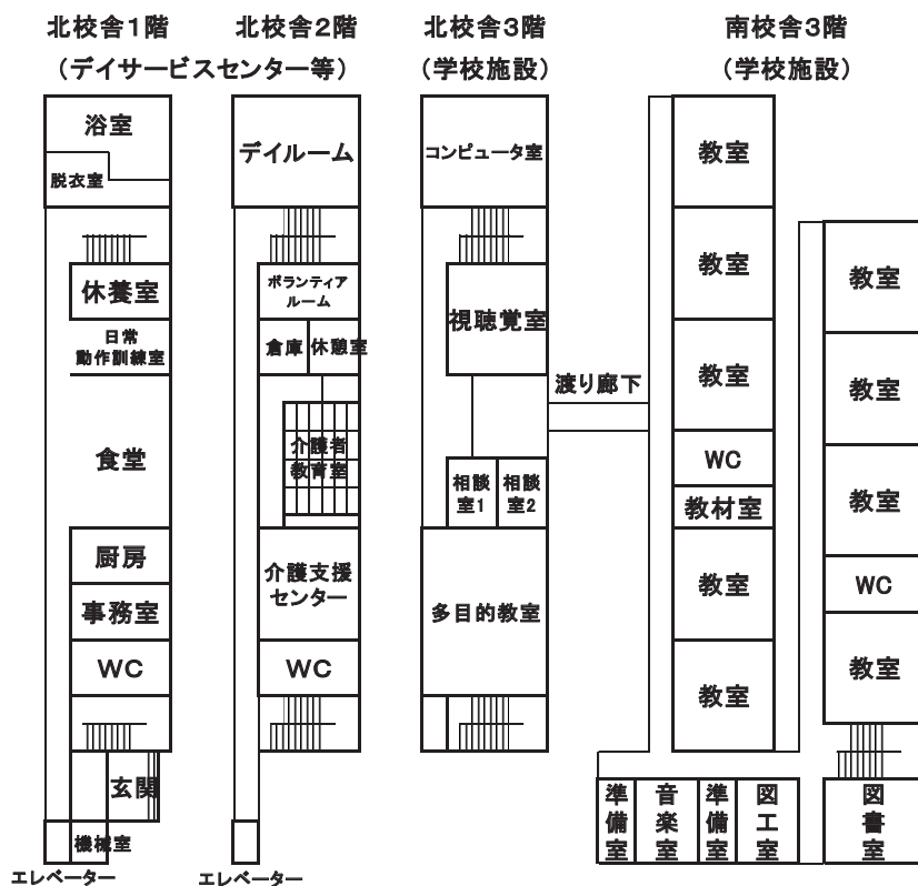
図2 小倉小学校の平面図
