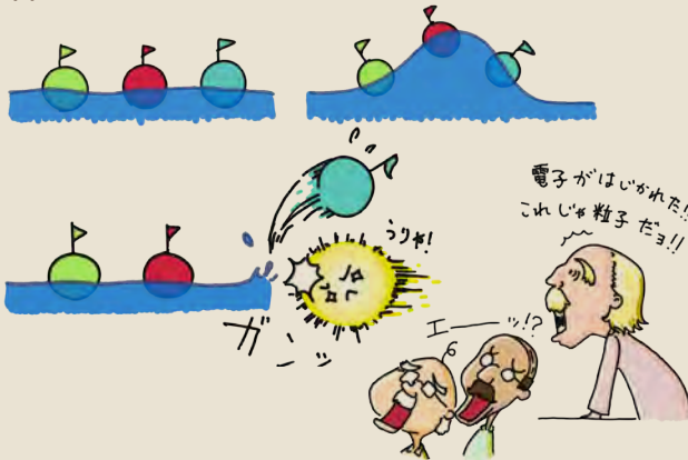
図A 光が波ならば全ての電子が動く
