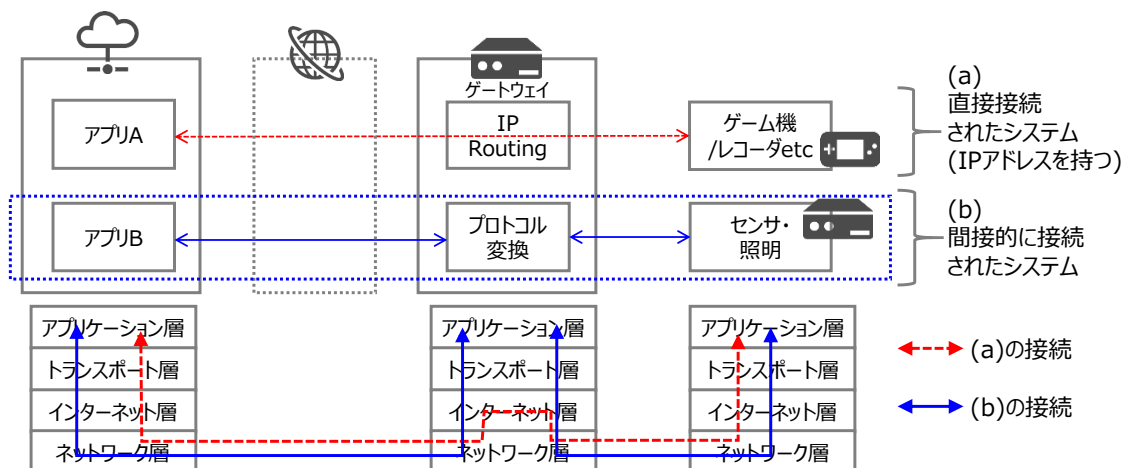
図 1-8 IoT システムのインターネット接続形態
