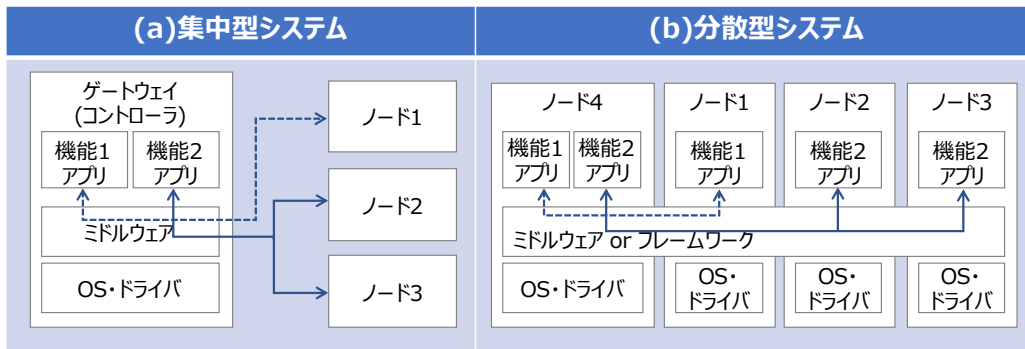
図 2-5 ネットワーク接続された組み込みシステムの構成とアーキテクチャ例
