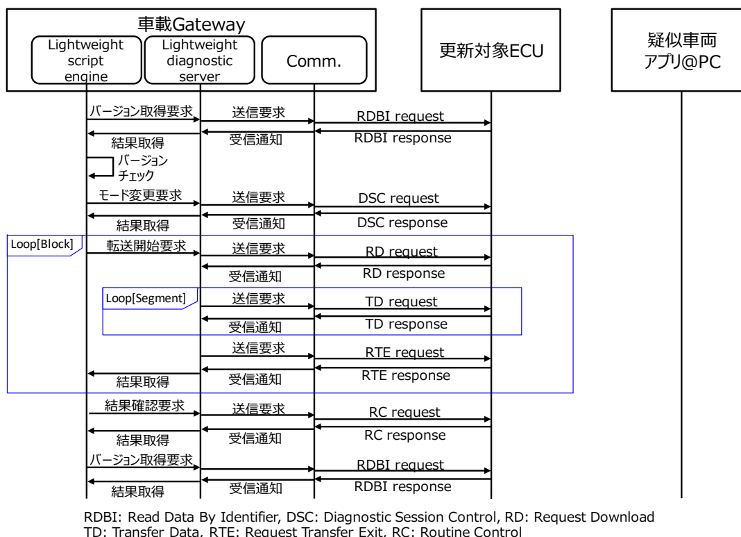
図 4-8 ECU 更新制御評価用更新シーケンス
