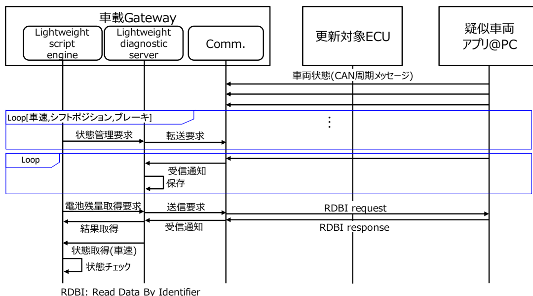
図 4-7 車両状態管理機能評価用更新シーケンス
