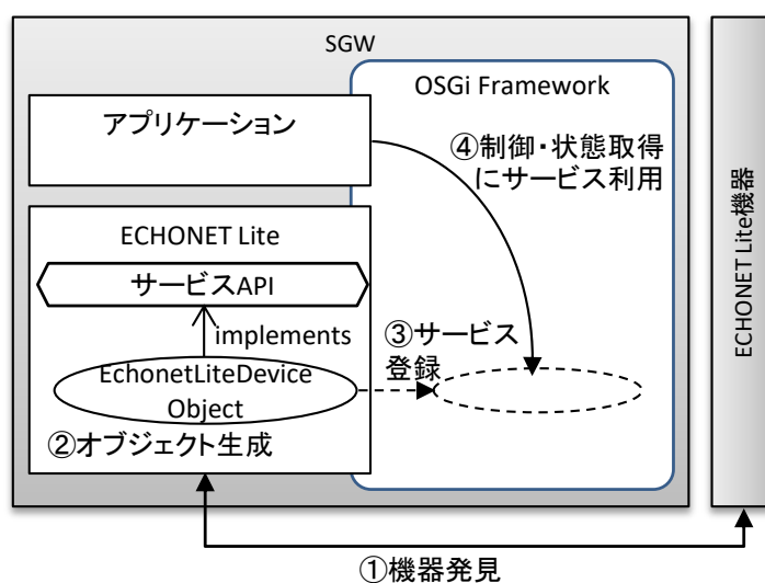
図 3-4 OSGi を利用した機器登録・利用方法
