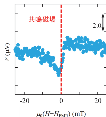
図2 非磁性電極から得られる起電力
