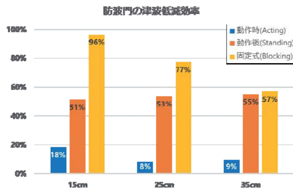
図-7.6 門式減勢工の津波減勢効果
