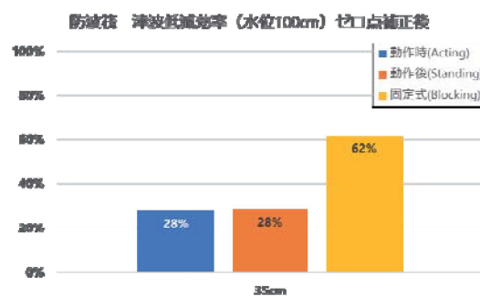
図-7.7 いかだ型減勢工の津波減勢効果
