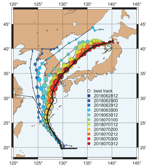
図 4.2 2018 年台風第 7 号の進路。太実線はベストトラック、その他は初期時刻を 2018 年 6 月 28 日 12 UTC から 7 月 3 日 12 UTC まで 12 時間間隔にして行った予報実験から作成。円が大きいほど中心気圧が低いことを示す。
