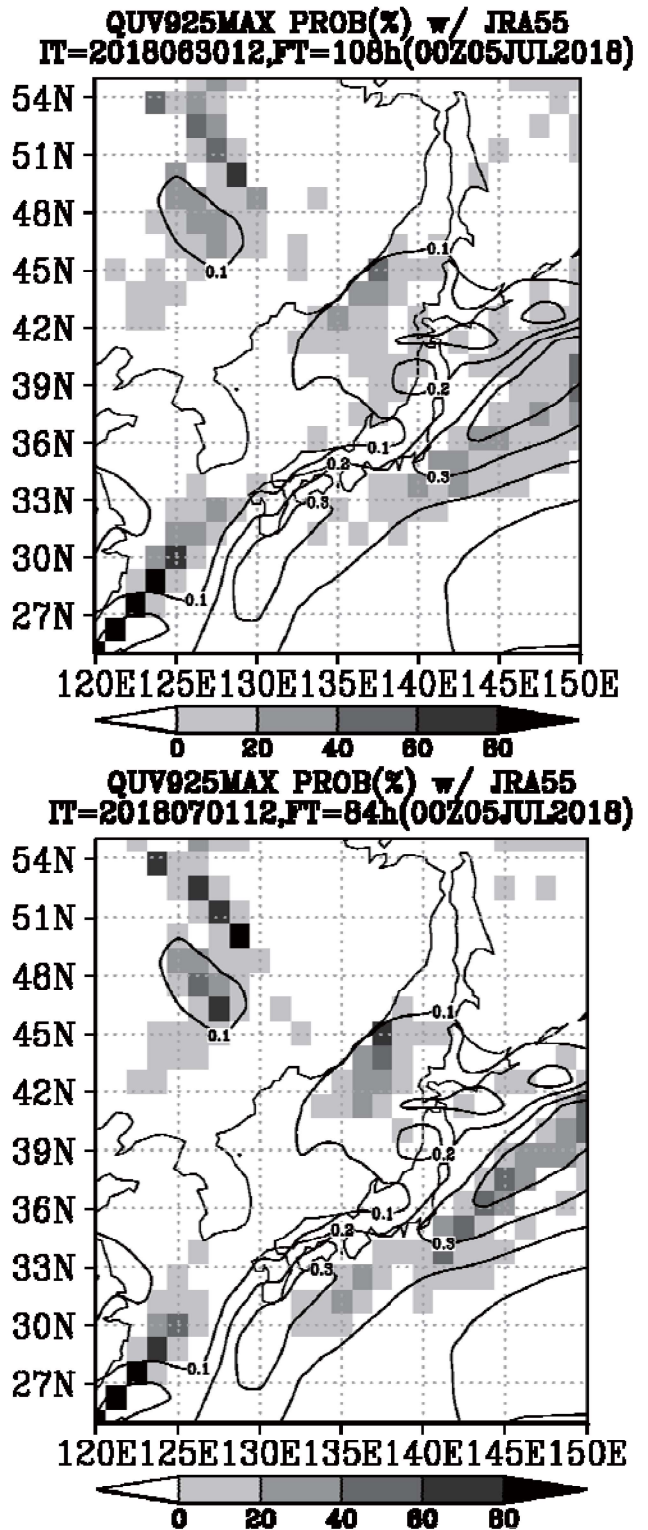
図 5.4 7 月 5 日 00UTC での 925hPa 水蒸気フラックス東西最大軸頻度分布 (陰影) と JRA-55 解析値 (黒線)。 (上) 6 月 30 日 12UTC 初期値, (下) 7 月 1 日 12UTC 初期値。
