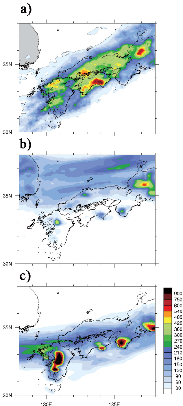
図 4.1 2018 年 7 月 5～7 日の 3 日間積算降水量 mm. a) 気象庁全国合成レーダー、初期時刻 2018 年 6 月 b) 28 日、c) 29 日 12 UTC からの予報実験
