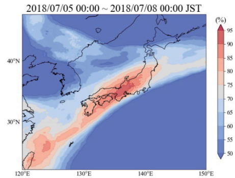
図3.7 700~300 hPaの鉛直層平均かつ時間平均した相対湿度場
