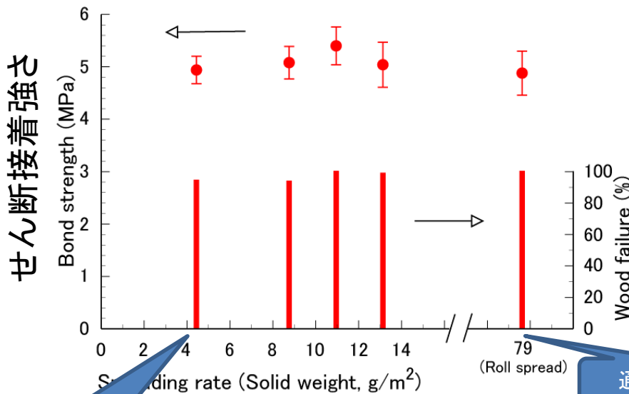
図2. 合板用フェノール樹脂の塗布量（横軸）と接着性能（縦軸）の関係
