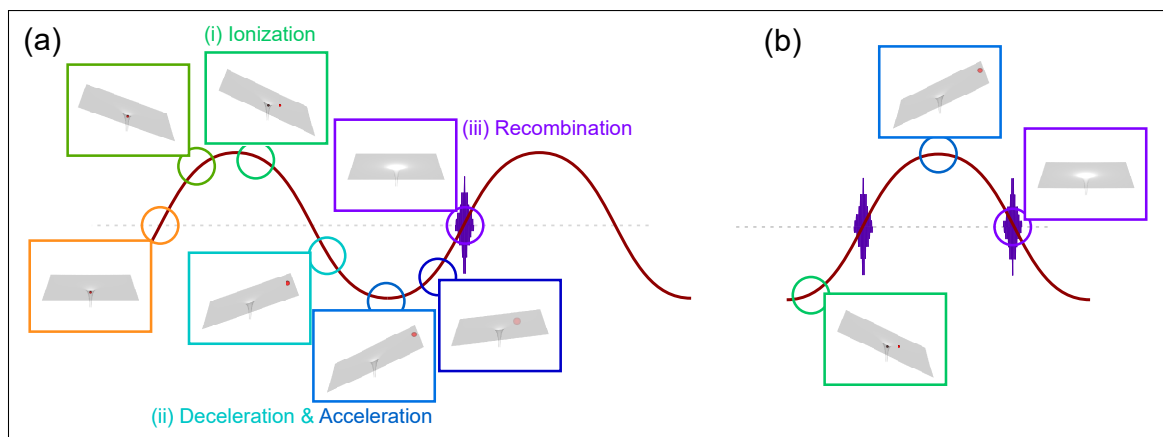
図 6 (a) ハーフサイクル内の 3 ステップモデル。(i) Ionization : 電子のイオン化、(ii) Deceleration & acceleration : 減速と再加速、(iii) Recombination : 再結合による光放射 (b) 3 ステップは各ハーフサイクルで繰り返すために、基本レーザーの半周期で繰り返される。
