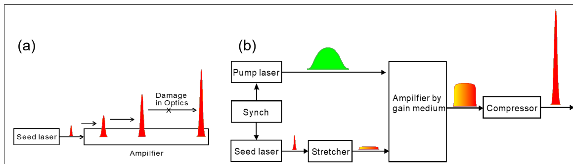
図 5 (a) 被増幅光をチャープさせないときのレーザー増幅。レーザー媒質の光破壊で高増幅率の達成は不可能である。(b) 被増幅光をチャープさせたときのレーザー増幅 (CPA)。シードレーザー (Seed laser) からの極短光パルスを時間的に伸ばし (Stretcher)、増幅後に時間的に圧縮 (Compressor) し、高強度フェムト秒パルスを得る。
