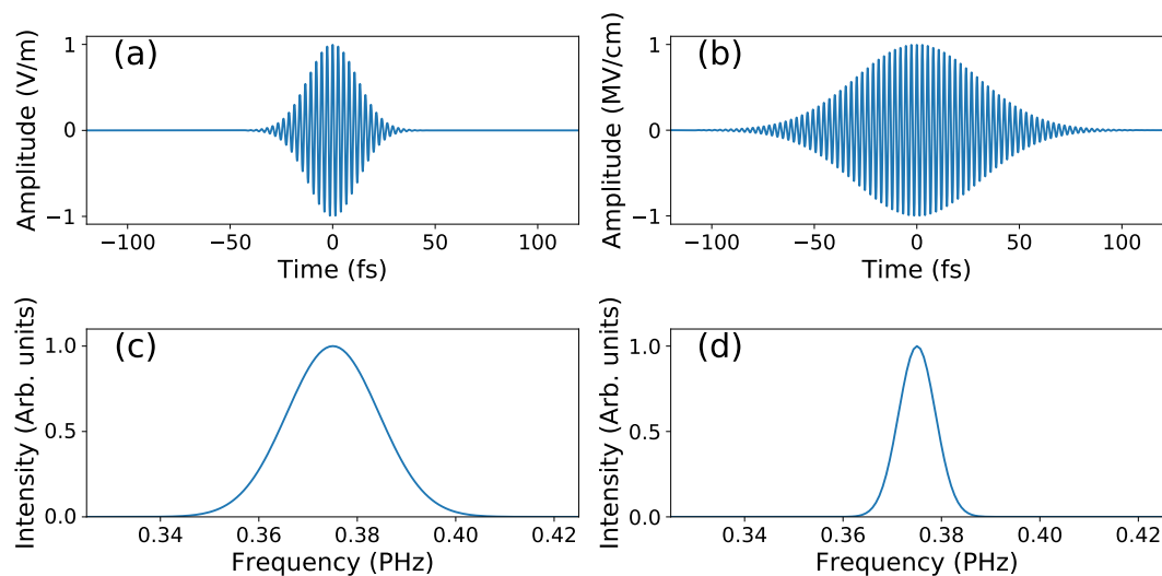
図 3 光電場パルスの時間幅とスペクトル幅の関係性
