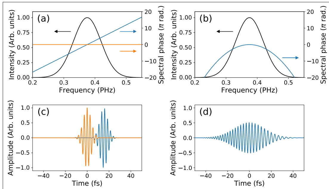
図4 光パルスとスペクトル位相の関係。(a) 共通したスペクトル強度（黒線）を用いて、スペクトル位相が零（オレンジ色）と周波数に対して線形な関係性を持つもの（青色）の2種類によって、それぞれ、電場波形が(c)のオレンジ線と青線になる。(b) スペクトル強度は(a)と同じであるが、位相が2次曲線にしたとき、電場波形は(d)のように時間的に伸長される。(d)の電場波形において、時間が負の時と正の時で振動の周期が変化していることに注目。
