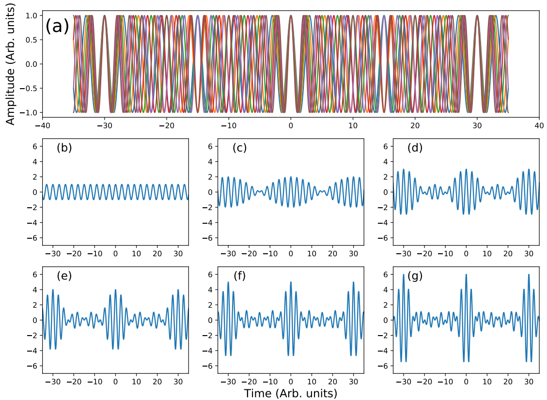
図2 (a) 最も低い周波数を f として、 1.1f 、 1.2f 、 1.3f 、 1.4f 、 1.5f の周波数を持つ合計 6 個の連続波。最低周波数の連続波 (b) に、順々に高い周波数の波を加えて重ね合わせた波形 (c) - (g)。
