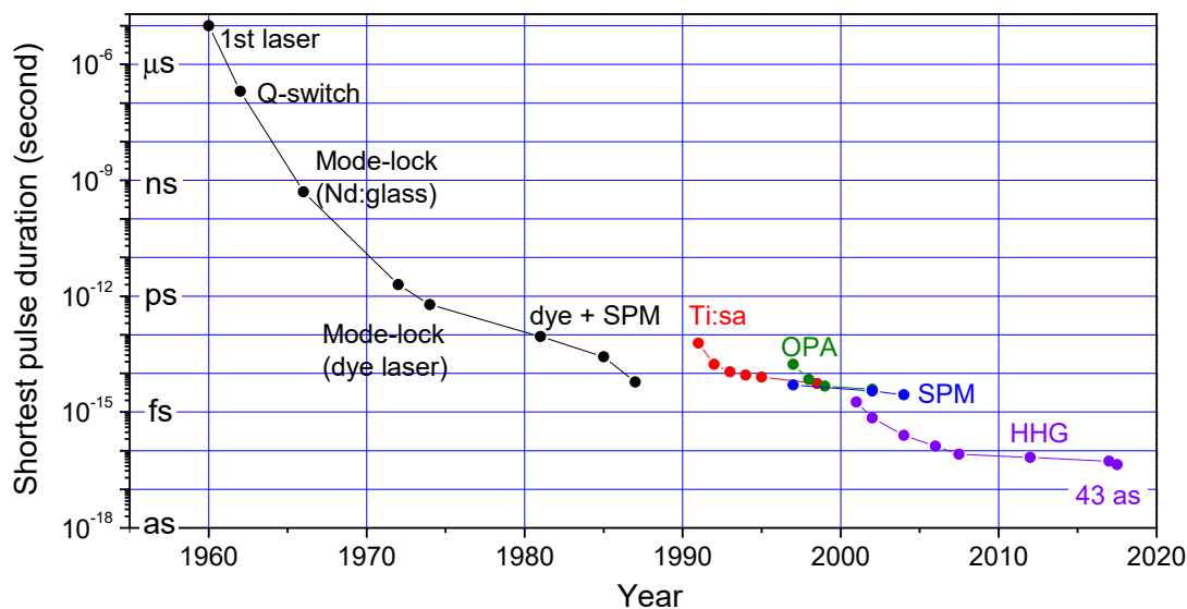
図8 光パルスの最短持続時間の変遷
