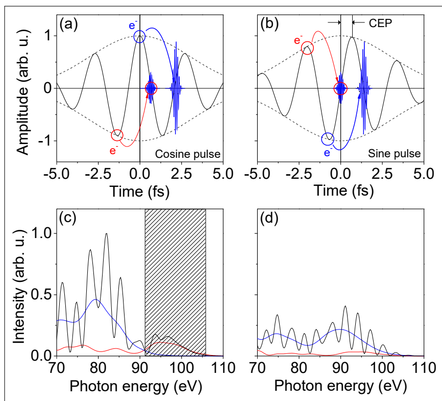
図7 2サイクル光パルスによるアト秒高調波発生。(a)、(c)は、それぞれ、コサインパルスの時の高次高調波発生電子軌跡と高次高調波のスペクトル。(b)、(d)は、それぞれ、サインパルスの時の高次高調波発生電子軌跡と高次高調波のスペクトル。網掛け部分が単一アト秒パルスのスペクトル領域であり、コサインパルスのみ発生が可能である。
