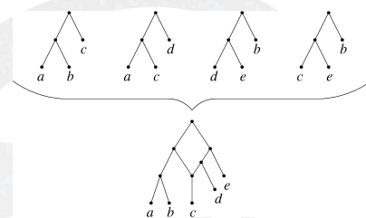
競合する系統樹セットから系統ネットワークを構築 Constructing a phylogenetic network from a set of conflicting phylogenetic trees.
