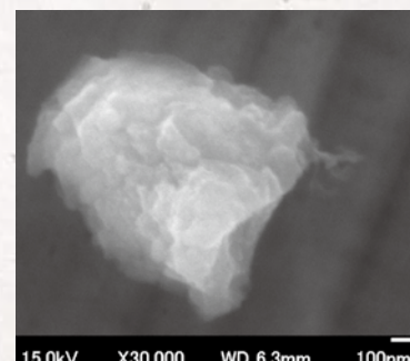
15.0kV X30,000 WD 6.3mm 100nm 太陽系形成前に漸近赤色分岐星で形成したプレソーラーコランダム (Al 2 O 3 ) 粒子。
