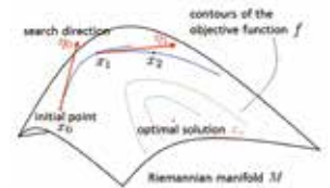
リーマン多様体上の最適化 Optimization on Riemannian manifolds
