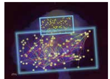
多ニューロン間での因果的な 相互作用ネットワーク Causal interaction networks among neurons
