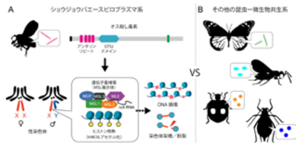
図2 共生細菌によるオス殺しの分子機構 (A) ショウジョウバエの共生細菌スピロプラズマが産生するオス殺し毒素のタンパク質構造 (上段)。二つの真核生物様ドメインを持つ。オス殺し毒素は、宿主オスの性染色体 (X染色体) だけに分布する遺伝子量補償複合体 (性分化機構の一つ) を足がかりにするらしい (下段左)。オスのX染色体に選択的に結合した毒素は、何らかの仕組みでDNA損傷や染色体の架橋・断裂を誘導し、オスのみを殺す (下段右)。(B) これまでに少なくとも6種のオス殺し共生細菌が報告されており、標的となる昆虫の種も多様である。性決定・分化の仕組みは昆虫種によって異なることから、未知のオス殺し毒素・機構の存在が示唆される。
