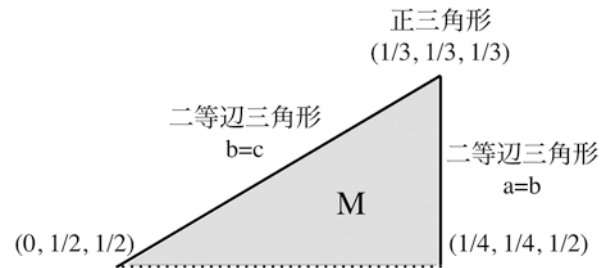
図1 三角形のモジュライ空間
