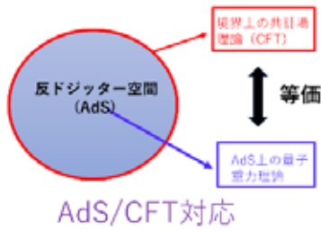
図1 AdS/CFT 対応概念図
