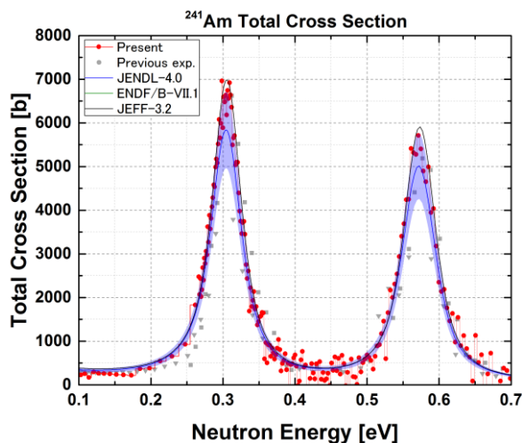
図 3. ^{241}\text{Am} の中性子全断面積
