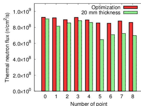
図 3. 最適化ボラスと 20mm 厚ボラス使用時の各評価点における熱中性子フラックス比較
