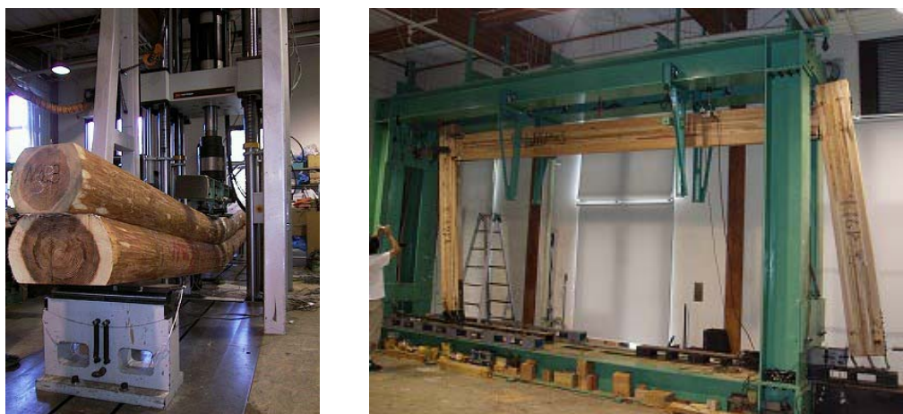
図 2.8 実大耐力実験装置
