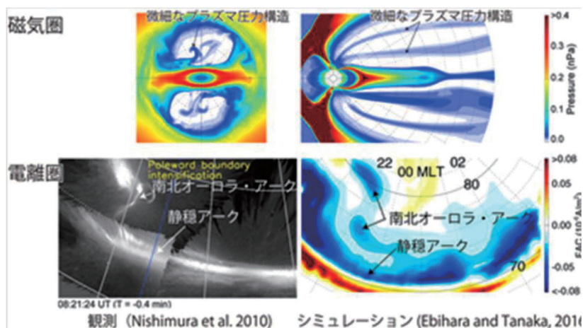
図3：オーロラ・アークのシミュレーション
