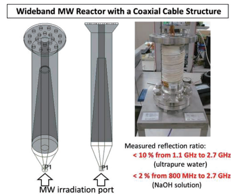
図7：化学反应用マイクロ波加熱容器の研究開発
