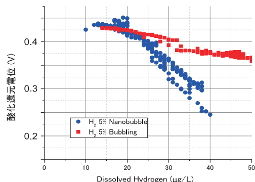
図4：微細気泡による溶存水素と酸化還元電位の相関
