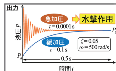
図3-2：加圧速度が圧力変化におよぼす影響（解析）
