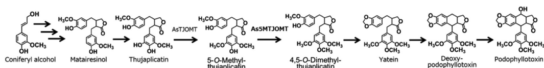
図1：シャクにおけるポドフィロトキシンの推定生合成経路
