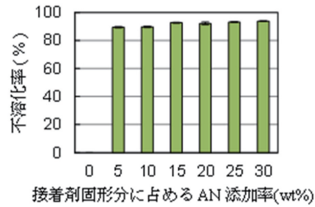
図2：AN 添加率が成形体の不溶化率に及ぼす影響
