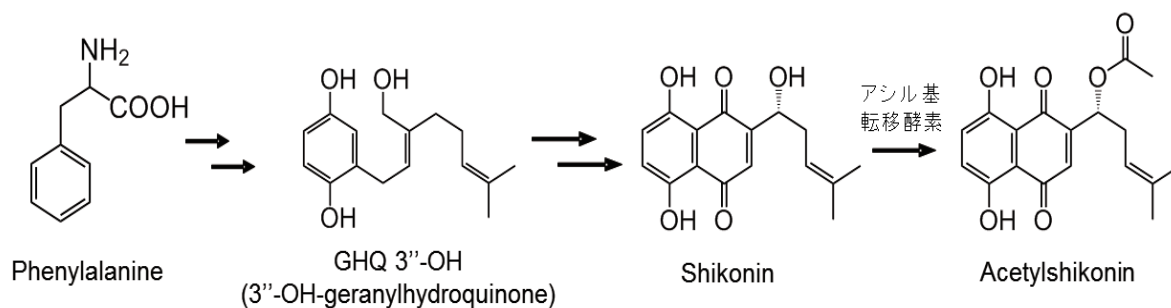
図1 シコニン類縁体生合成経路
