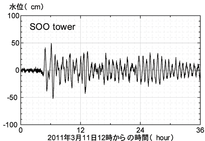
図 2 田辺中島高潮観測塔での津波波形
