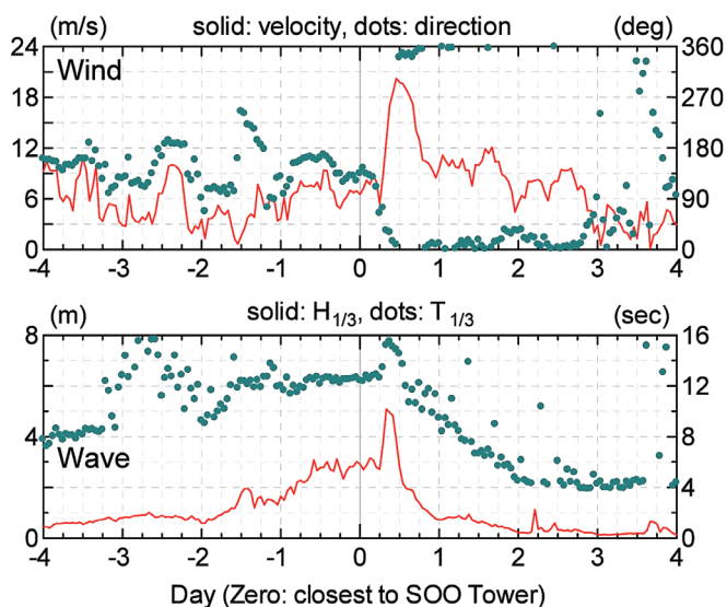
(b) 台風 15 号接近時
