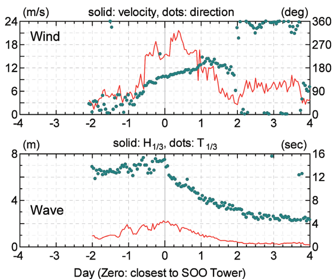
(a) 台風 12 号接近時
