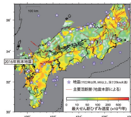
GNSS観測によって得られた西南日本における2005-2009年の最大せん断ひずみ速度。南海トラフのプレート間固着による影響は補正した
