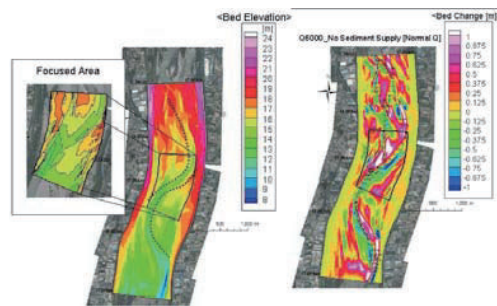
アユの産卵床に適した河床地形の評価・予測のための研究例 Studies for evaluation and prediction of geomorphology suitable for spawning sites of Ayu fish
