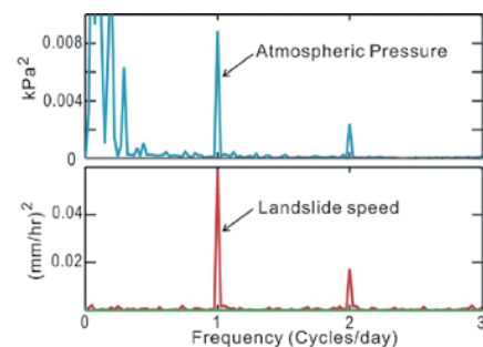
気圧変動にシンクロする地すべりの変動 (コロラド州、USA) Air tides and landsliding: power spectra of atmospheric pressure and landslide speed for Slumgullion landslide, Colorado, USA
