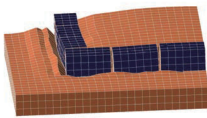
左：2011年東北地方太平洋沖地震・津波で被災した岸壁 Left : Damaged quay walls after the 2011 Off the Pacific coast of Tohoku earthquake 右：重力式岸壁の3次元有限要素法による変形シミュレーション Right : 3D simulation of gravity quay walls during earthquakes
