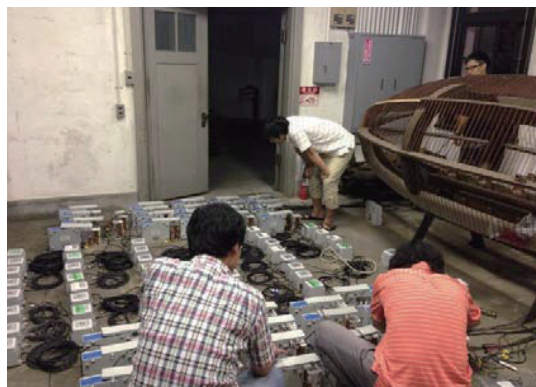
稠密観測（満点計画）用の小型地震計の整備 Portable seismometers for the dense array observations
