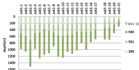
大阪平野南部における常時微動の水平上下スペクトルから同定した地下構造モデル Subsurface structure of the southern part of Osaka plain identified from Horizontal-to-Vertical spectral ratio of microtremors
