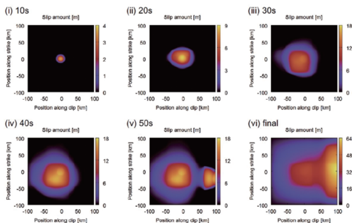
東北地方太平洋沖地震の動的破壊シミュレーション（TPを考慮） Dynamic rupture simulation for the 2011 Tohoku Earthquake considering the effect of thermal pressurization
