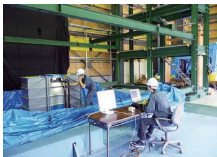
強震応答実験室の大型振動台での実験 Vibration test by three dimensional shaking table
