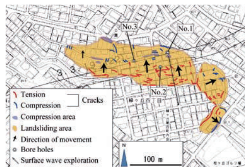
2011年東北地方太平洋沖地震による仙台市住宅地の地すべり Landslide in urban residential fills caused by the 2011 Tohoku earthquake
