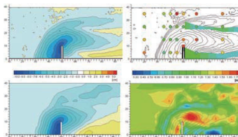
混合砂を用いた水制周辺の地形変動（左）および河床材料の粒度変化（右）に関する実験結果（上）およびシミュレーション結果（下） Change of river bed topography (left) and bed material size (right) around the groyne and their experimental results (above) and simulation results (below)
