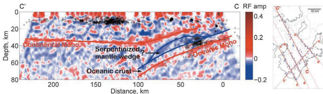
CC'測線（尾鷲～京丹後測線）に沿う断面における地震波速度不連続面の形状。紀伊半島下に沈み込むフィリピン海プレートがイメージされている。 Seismic wavespeed discontinuity in a cross section along the profile line CC'. The Philippine Sea plate subducting beneath Kii Peninsula is clearly imaged.
