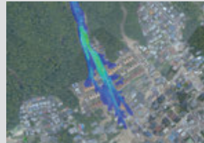
2014年8月に広島市安佐南区八木三丁目で発生した土石流の氾濫の様子の数値解析 Numerical simulation of debris flow inundation which occurred in Hiroshima, 2014
