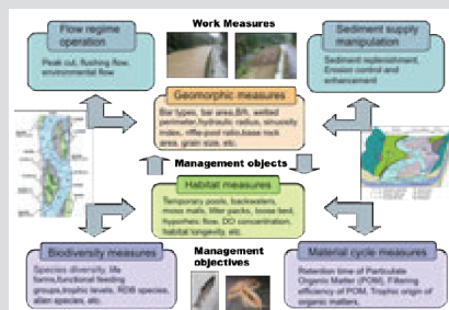
統合的流域管理のための河床地形管理手法の開発図式 Conceptual framework of the riverbed geomorphology management for integrated basin management
