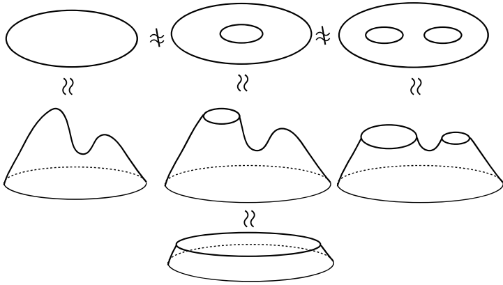
図 4. 円板 \not\approx 円環 \not\approx パンツ
