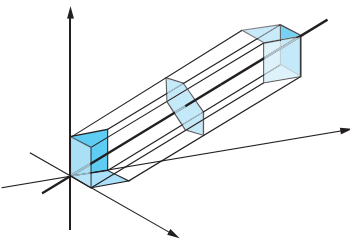
図 2: \mathbb{L}^1 凸集合 P = \{p \in \mathbb{Z}^3 \mid (0, 0, 0) \leq p \leq (12, 12, 12), p_j - p_i \leq 3 \ (1 \leq i, j \leq 3, i \neq j)\} の凸包. その中心を対角線 \{(z_1, z_2, z_3) \in \mathbb{Z}^3 \mid z_1 = z_2 = z_3\} が貫く.
