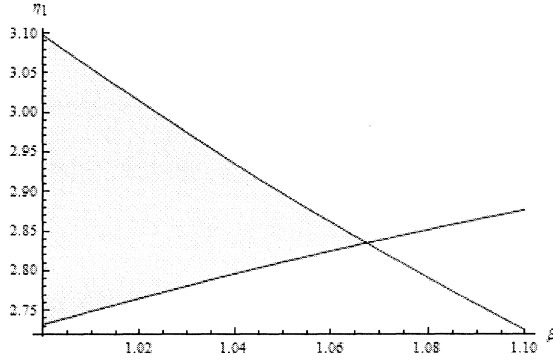
図 6: Non ergodic parameters
