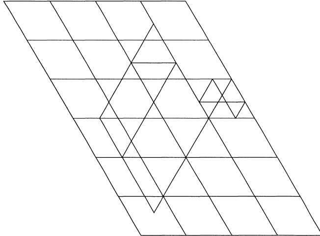
図 8: 3-fold sofic case
