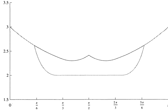
図 7: B_1 と B_2 の比較
