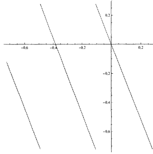
図 2: 負のベータ展開 \beta = 2.6
