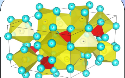
アパタイトの結晶構造
