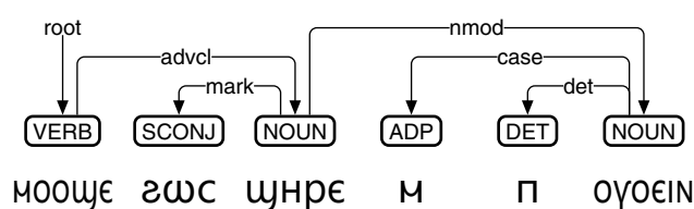
図 105: roberta-base-coptic-upos によるコプト語の係り受け解析
