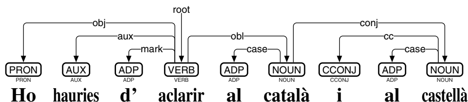
図 118: Trankit によるカタルーニャ語の係り受け解析
