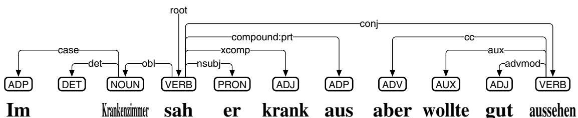
図 57: ドイツ語向け品詞付与・係り受け解析ミニモデルのテスト
