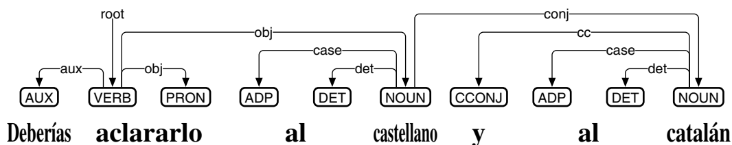
図 112: Stanza によるスペイン語の係り受け解析
