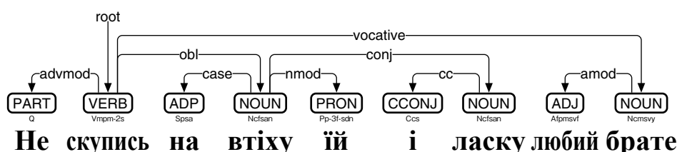
図 78: Trankit によるウクライナ語の係り受け解析
