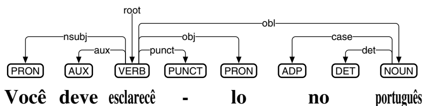
図 137: ポルトガル語向け品詞付与・係り受け解析ミニモデルのテスト
