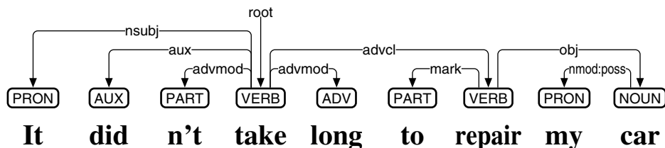
図 43: 英語向け品詞付与・係り受け解析ミニモデルのテスト
