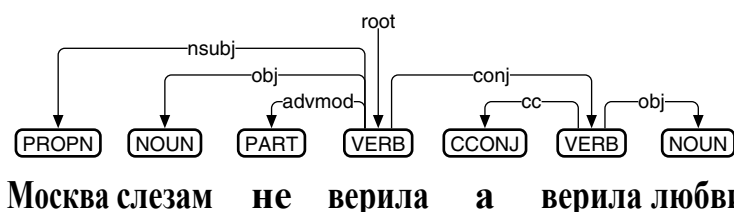
図 77: ロシア語向け品詞付与・係り受け解析ミニモデルのテスト
