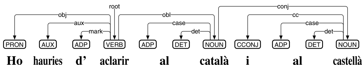
図 119: Stanza によるカタルーニャ語の係り受け解析
