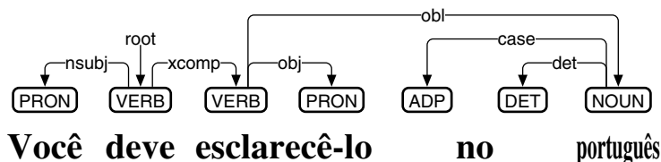
図 132: UDPipe 2 WebAPI によるポルトガル語の係り受け解析
