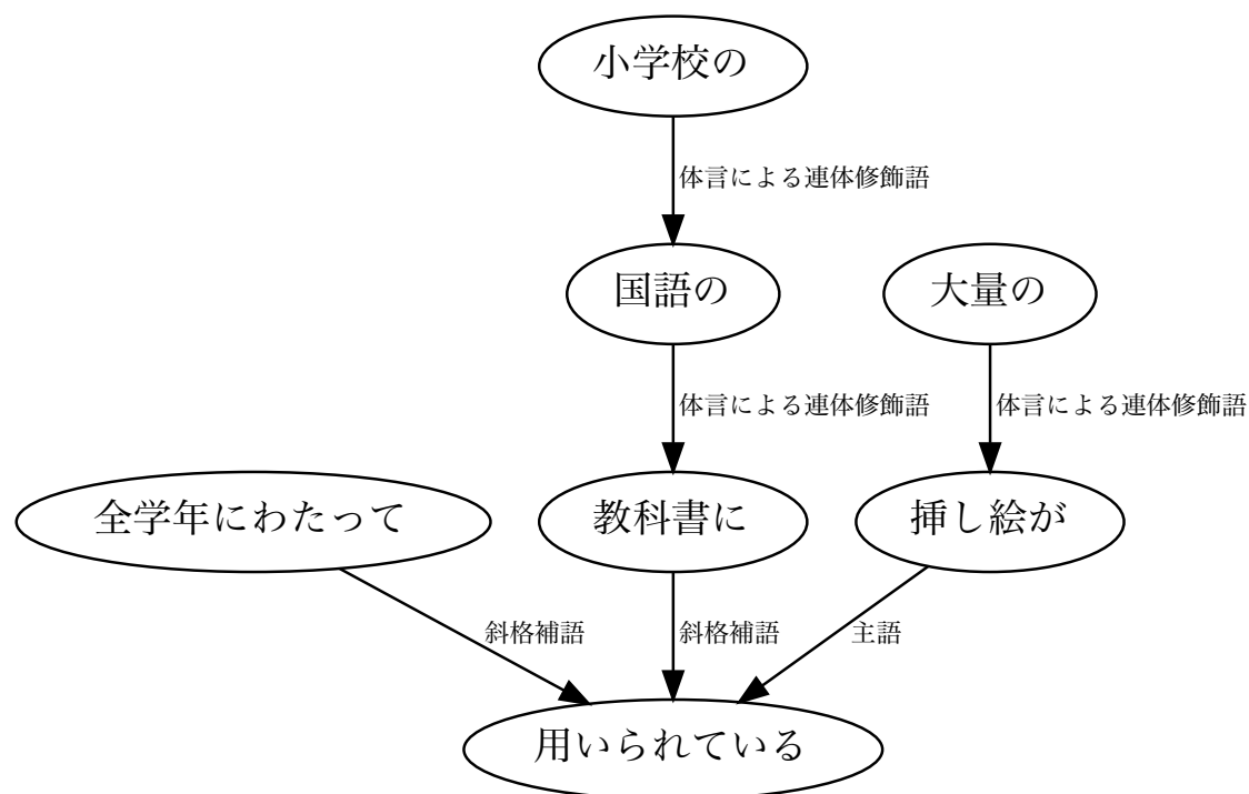
図 36: 文節にもとづく日本語係り受け解析
