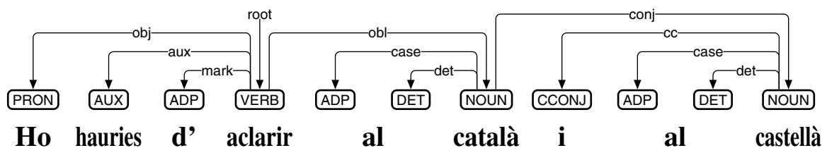
図 124: カタルーニャ語向け品詞付与・係り受け解析ミニモデルのテスト
