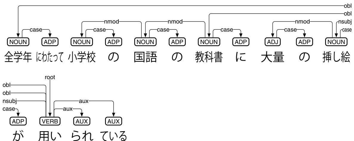
図 33: roberta-base-japanese-luw-upos による日本語係り受け解析 (国語研長単位)
