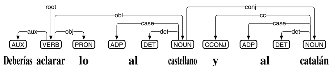
図 117: スペイン語向け品詞付与・係り受け解析ミニモデルのテスト
