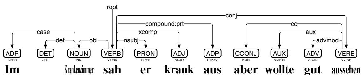
図 52: Trankit によるドイツ語の係り受け解析
