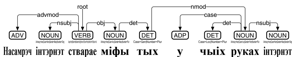
図 84: Camphr-Udify によるベラルーシ語の係り受け解析
