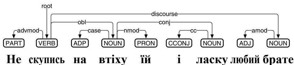
図 83: ウクライナ語向け品詞付与・係り受け解析ミニモデルのテスト
