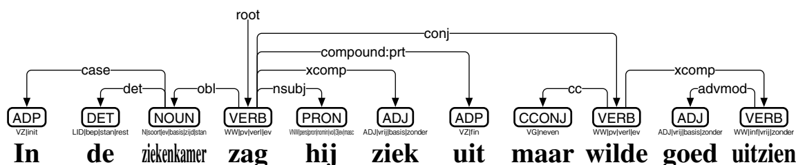
図 59: Trankit によるオランダ語の係り受け解析
