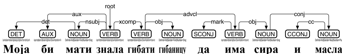
図 90: Camphr-Udify によるセルビア語 (キリル文字) の係り受け解析
