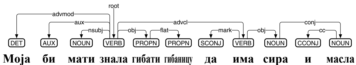
図 97: セルビア語向け品詞付与・係り受け解析ミニモデルのテスト
