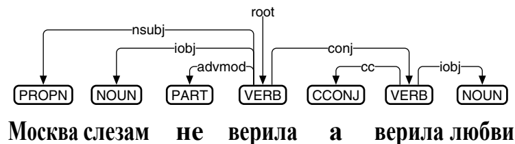
図 72: Trankit によるロシア語の係り受け解析
