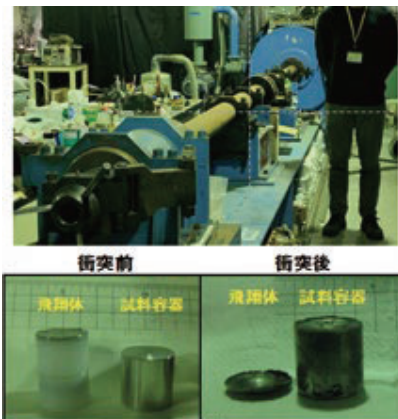
図2. 一段式火薬銃と衝突前後の飛翔体・試料容器
