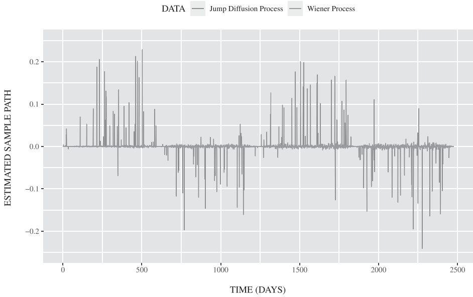
図 4 : \Lambda_{je}(t) の場合における推定された N_w(t) および N_j(t) のサンプルパス.
