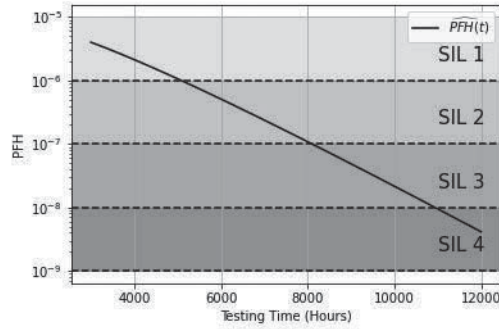
図 3： 推定された PFH の挙動.
