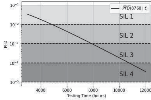
図 2： 推定された PFD の挙動.
