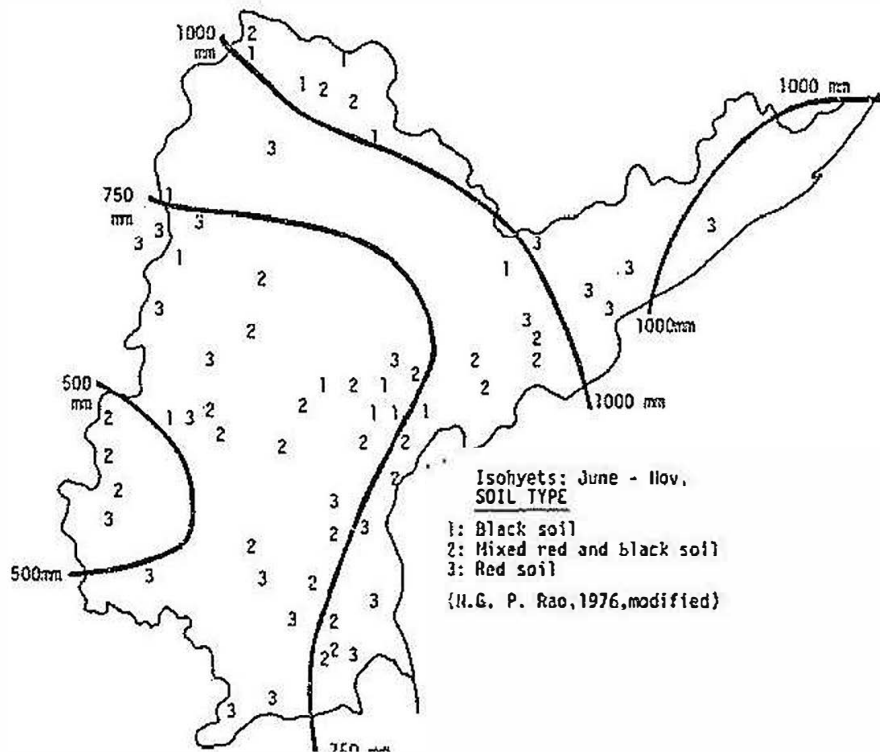
第4図 アンドラプラデシュ州のカリフ(雨季)降水量と土壌型の分布 (N.G.P. Rao, 1976を一部変更)
