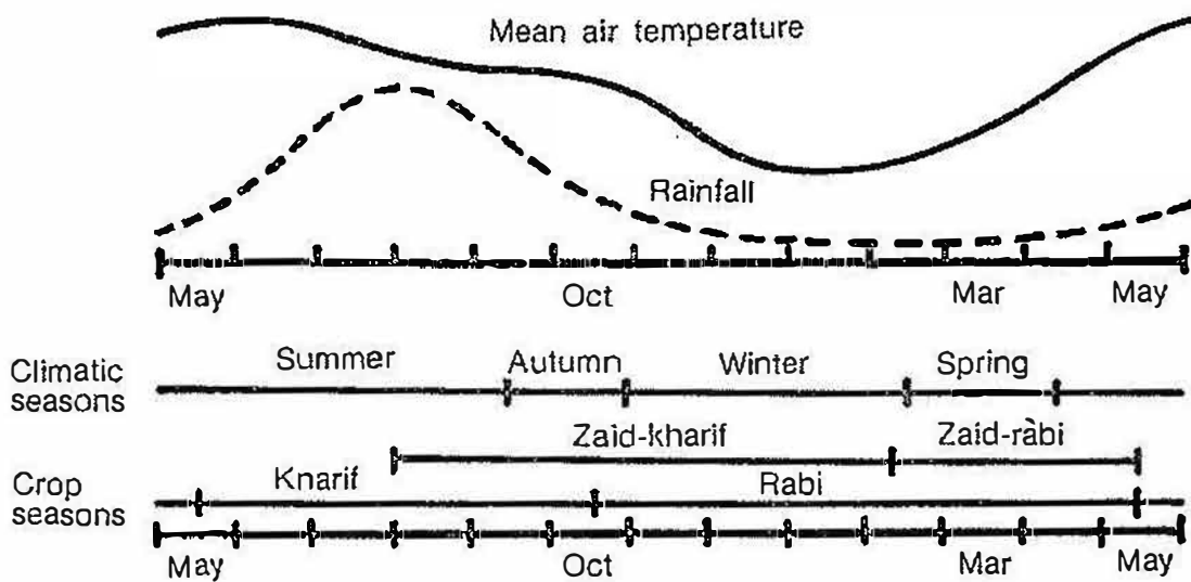
第3図 インドにおける降水量と気温の年変化パターンと作季との関係概念図 (前田1977) (Indian Crop Calender, I.C.A.R., 1967により作図)
