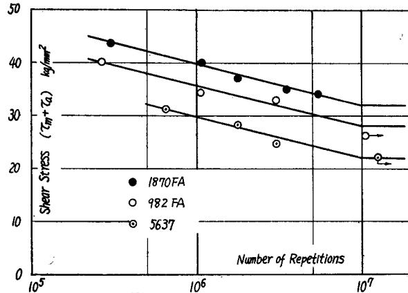
Fig. 11. S-N diagram.
