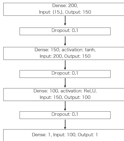
図 6： 深層学習モデルの構造。
