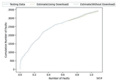
(b) SWC.
