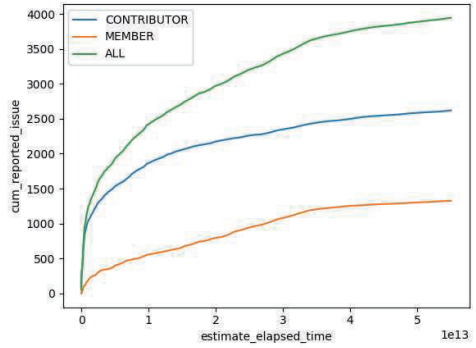
(d) vite.
