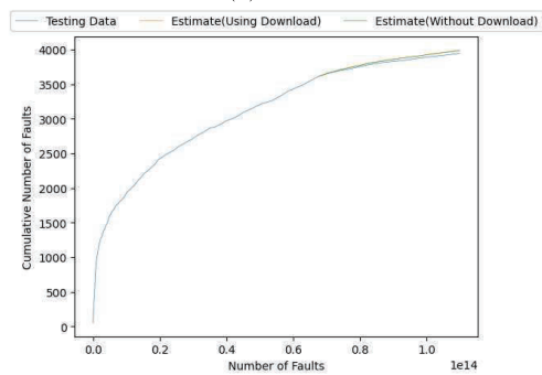
(d) vite.
