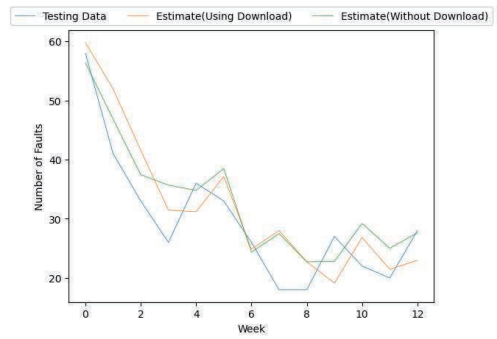
(d) vite.
