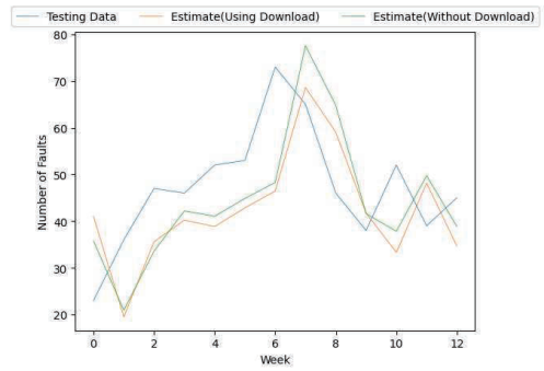
(b) SWC.
