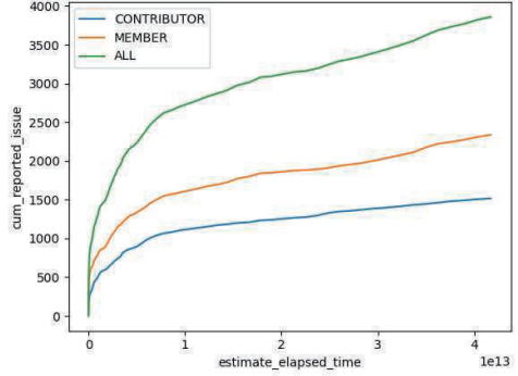
(b) SWC.
