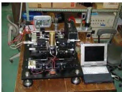
Figure 8 応力測定装置
