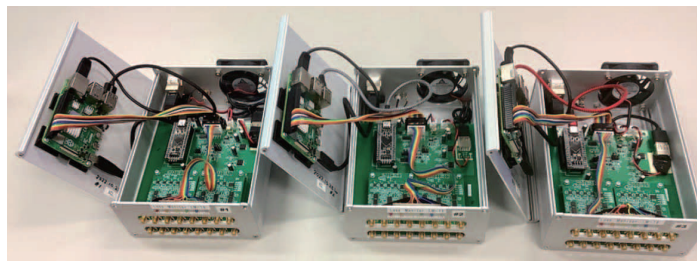
Raspberry Piを制御に使用したビームロスモニタの読み出し系
