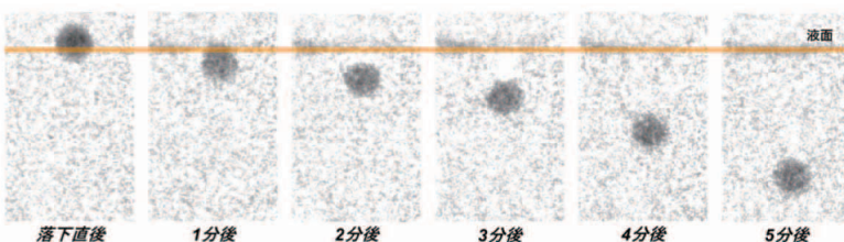
図. 溶けた液体ガラスの中を落ちていく金属球の様子を中性子で視た結果
