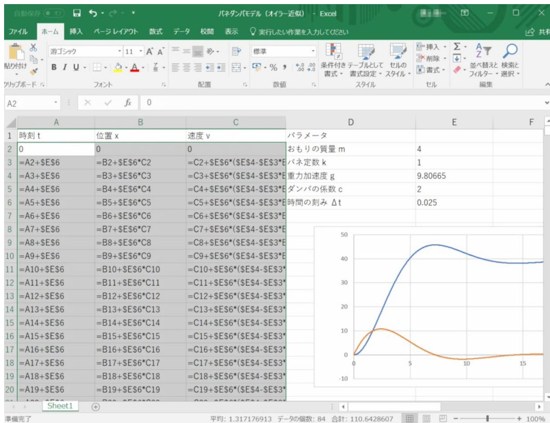
図 77 バネ・ダンパモデルのシミュレーション
