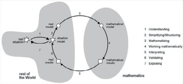
図 2: 数理モデリング・サイクル [4]
