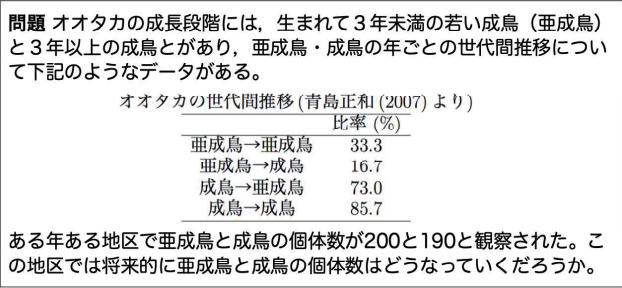
図 5: 問題例 (2): オオタカの個体数推移 ([16, p.159], [2])
