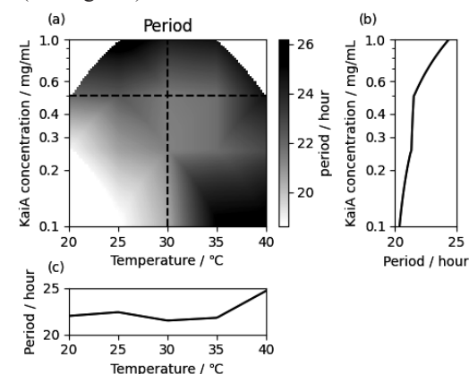
図3. (a) リン酸化度の振動周期の KaiA 濃度および温度依存性。各測定点間は線形に内挿した。(b), (c) はそれぞれ(a)内に点線で示した温度 (30°C) と KaiA 濃度 (0.5 mg/mL) での振動周期を示す。
