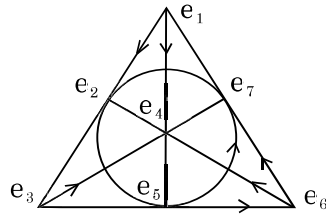
図1 八元数の積
