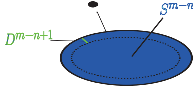
Figure 1: Proposition 1 で、special generic 写像 f からでてくる商写像 q_f : M \rightarrow W_f の値域の多様体 W_f といくつかの点や線分の逆像。例えば W_f の境界上の点の逆像は 1 点集合である。
