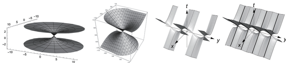
図 1. 楕円的カテナイド (左端), 放物的カテナイド (中央左), 双曲的カテナイド (中央右) と双曲的カテナイドの像の解析的拡張 (右端)
