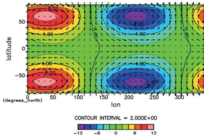
図 10: 角運動量輸送に最も貢献している波動 (帯状波数 1, 振動数 0.432 [ \text{day}^{-1} ]) の水平構造. \gamma = 1 の場合. 高度 784 Pa での水平風 (矢印) とジオポテンシャル高度 (等値線) を示している. 赤色と青色がそれぞれ高気圧と低気圧に対応する (Sumi et al., 2022).
