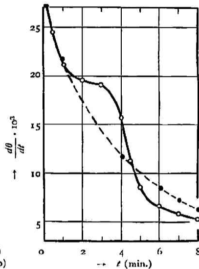
Fig. 15.—Expt. 15. (O: obs.; ●: calc.)
