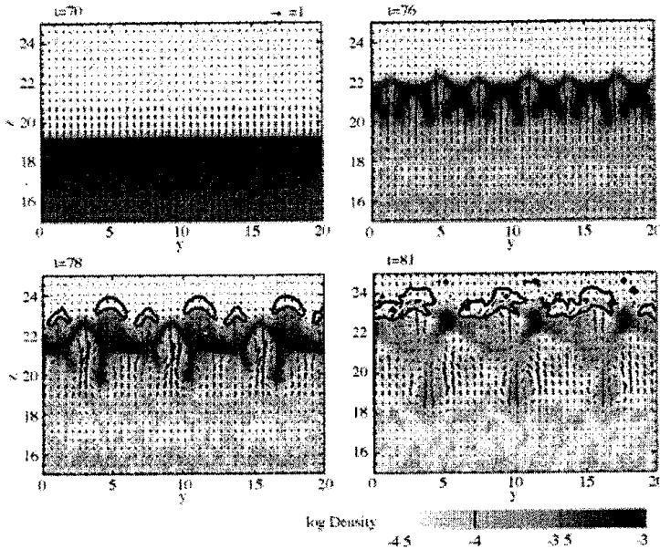
図 3 浮上磁場中央部分の密度（グレイコントラスト）と速度場（矢印）の時間発展。太い実線のコントラストは異常抵抗の分布を示す。磁場は紙面に垂直。
