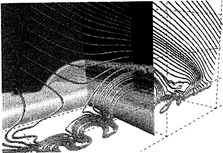
図 2 3 次元シミュレーションの結果。磁力線と断面の密度分布を示す。密度は色が明るい方が密度が高い。
