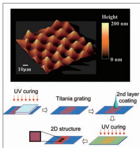
図2 自己組織的に形成した二次元フォトニック構造チタニア薄膜の原子間力顕微鏡像。周期構造チタニア薄膜を基板上に形成し、第二層を同様のプロセスで形成する。第二層は第一層に垂直に周期構造を形成するために二次元フォトニック構造を非常に簡単に得ることができる。上図は、励起光として市販のブラックライト、シリカガラス基板とコーティング液のみで形成することが可能であり、簡便な大面積フォトニック構造形成手法として注目される。
