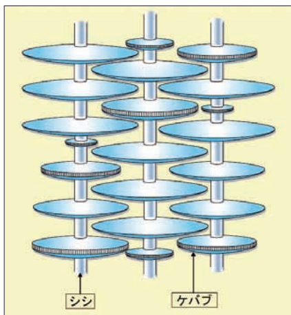
図1 シシケバブの模式図。 シシ：伸張鎖結晶、ケバブ： 折り畳み鎖ラメラ晶。
