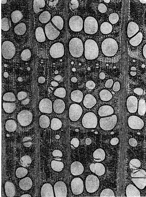
木口 (×25)
