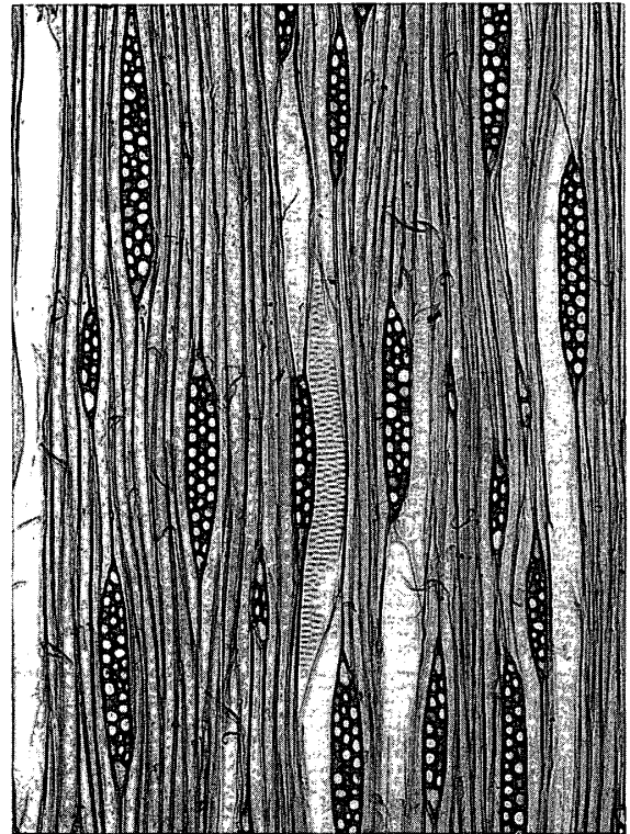
板目 (×80)
