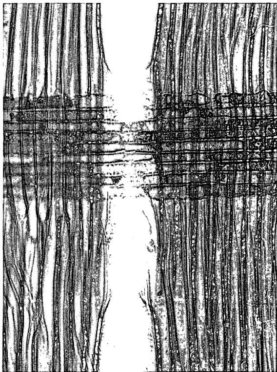
柁目 (×200)
