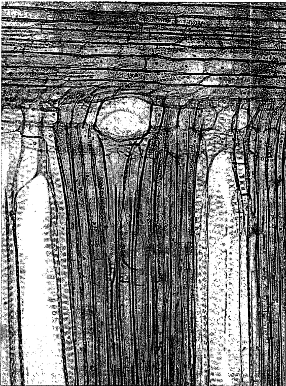
柁目 (×160)
