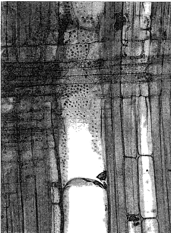
柎目 (×200)
