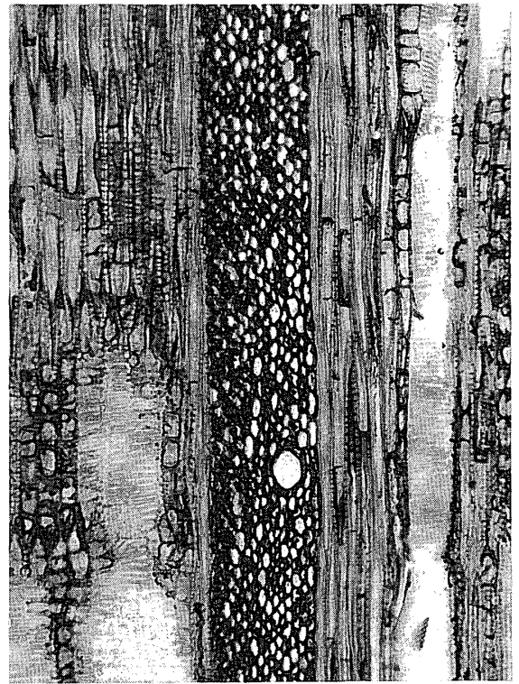
板目 (×50)
