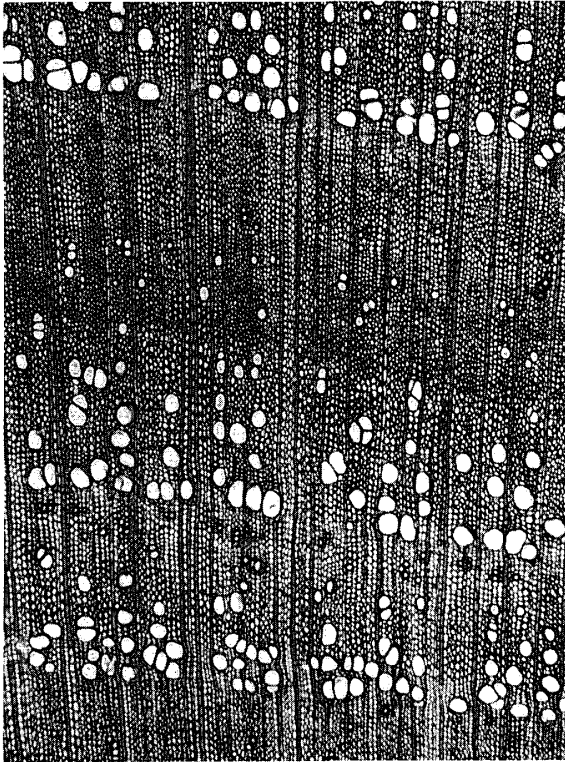
木口 (×25)
