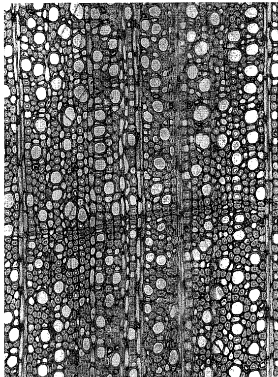
木口 (×100)
