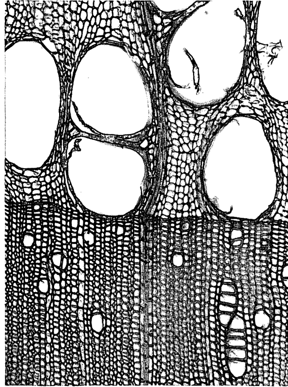
木口 (×100)
