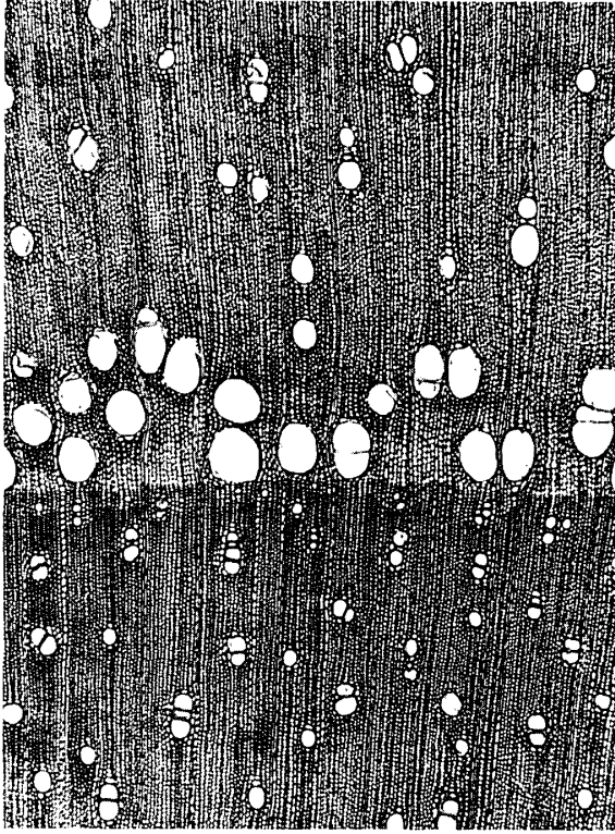
a 木口 (×25)
