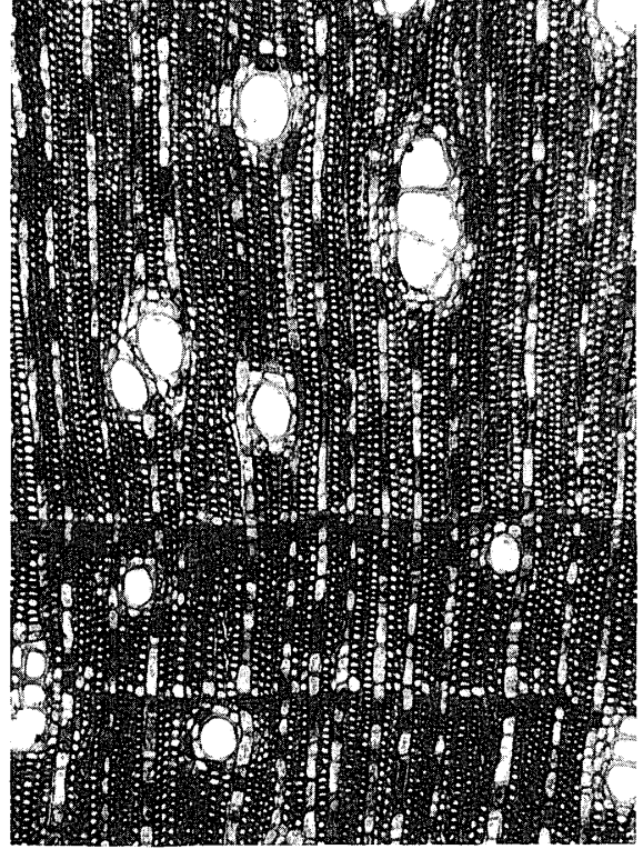
木口 (×80)
