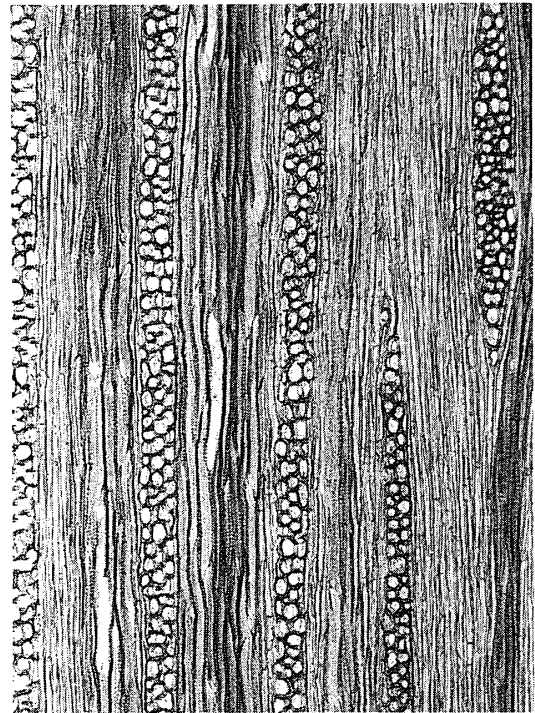
板目×80
