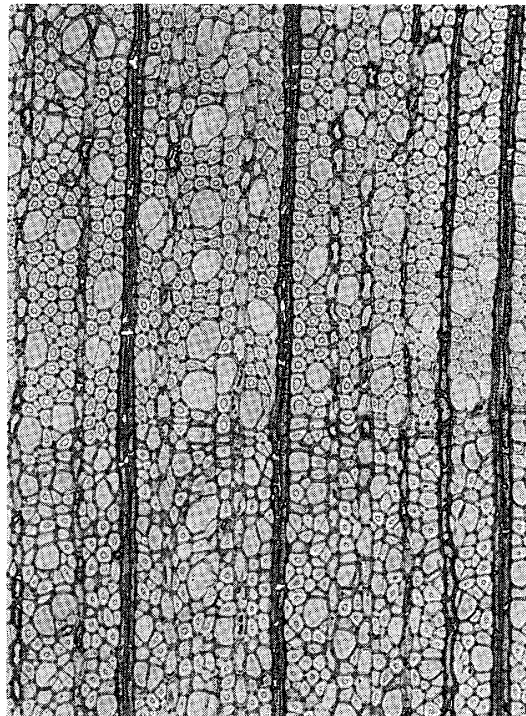
木口×100
