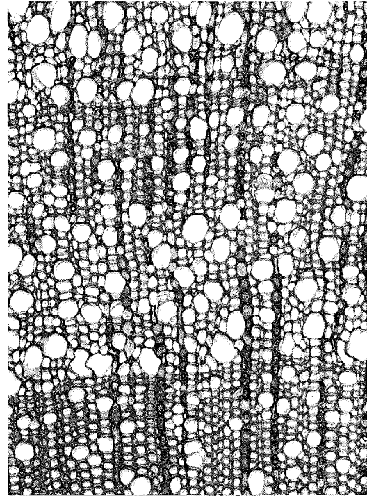
木口×160
