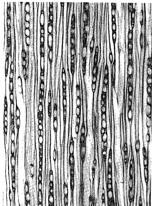
板目×130
