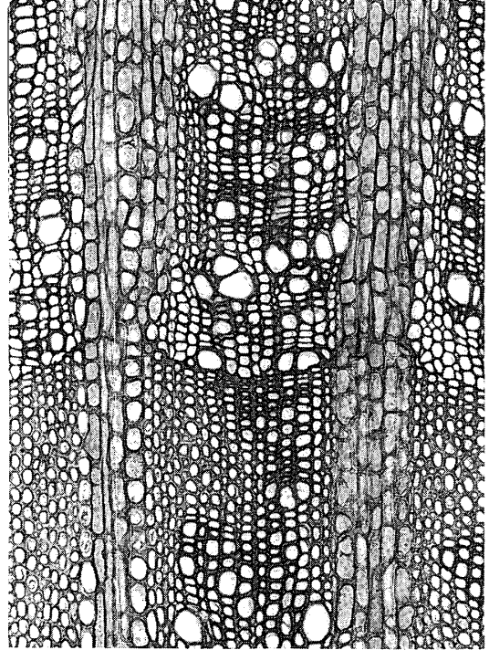
木口×130
