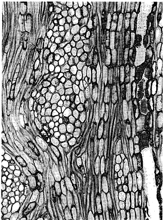
板目×130
