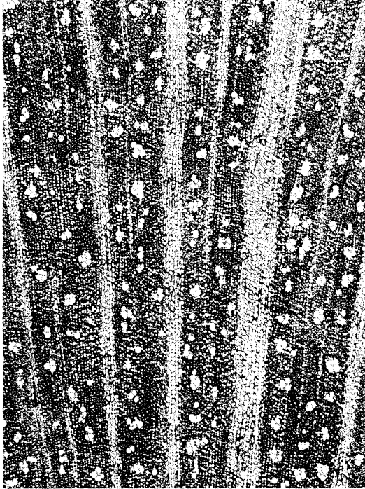
木口×25
