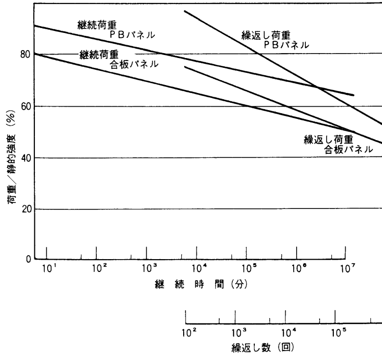
図7 疲労及びクリープ破壊における繰返し荷重/静的強度—繰返し数，継続荷重/静的強度—継続時間の関係
