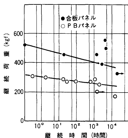
図5 クリープ破壊における継続荷重—継続時間の関係
