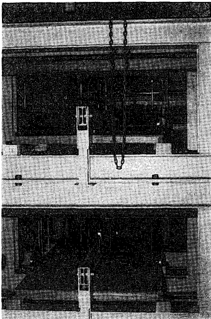
写真1 クリープ試験装置 手前が荷重のためこの支点、スペースの有効利用のため試験装置を上下に2・3段積重ねることができる。
