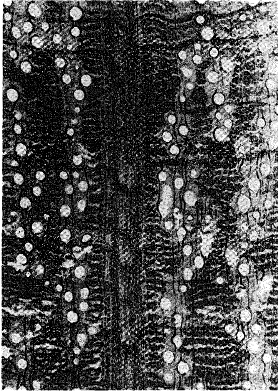
図7 (木口面) テコ ×15
