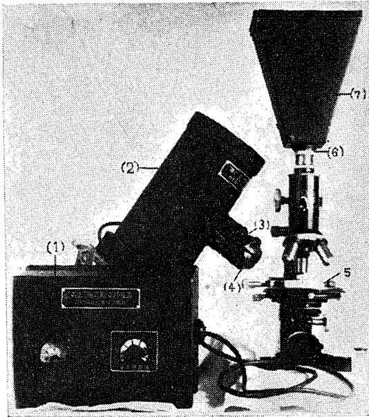
(1) 変圧器 (2) ランプ室 (3) wood氏フィルター (4) 集光レンズ (5) 試片 (6) 4%フィルター (7) 暗箱
